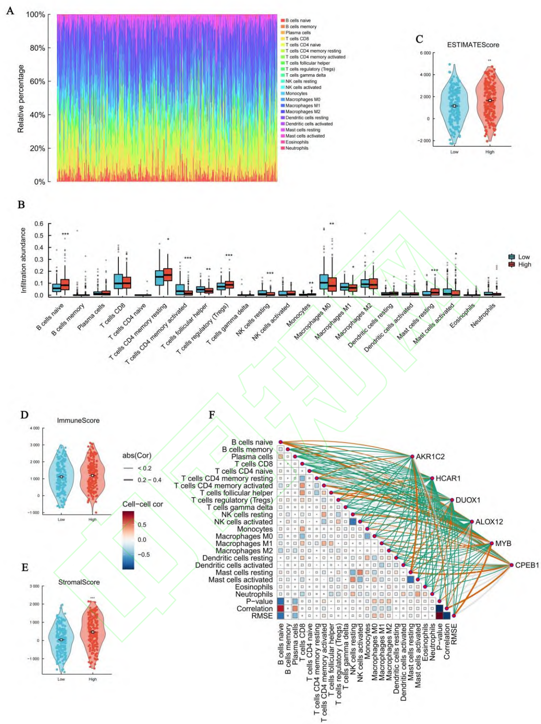
图 4 胃癌患者免疫浸润情况分析
