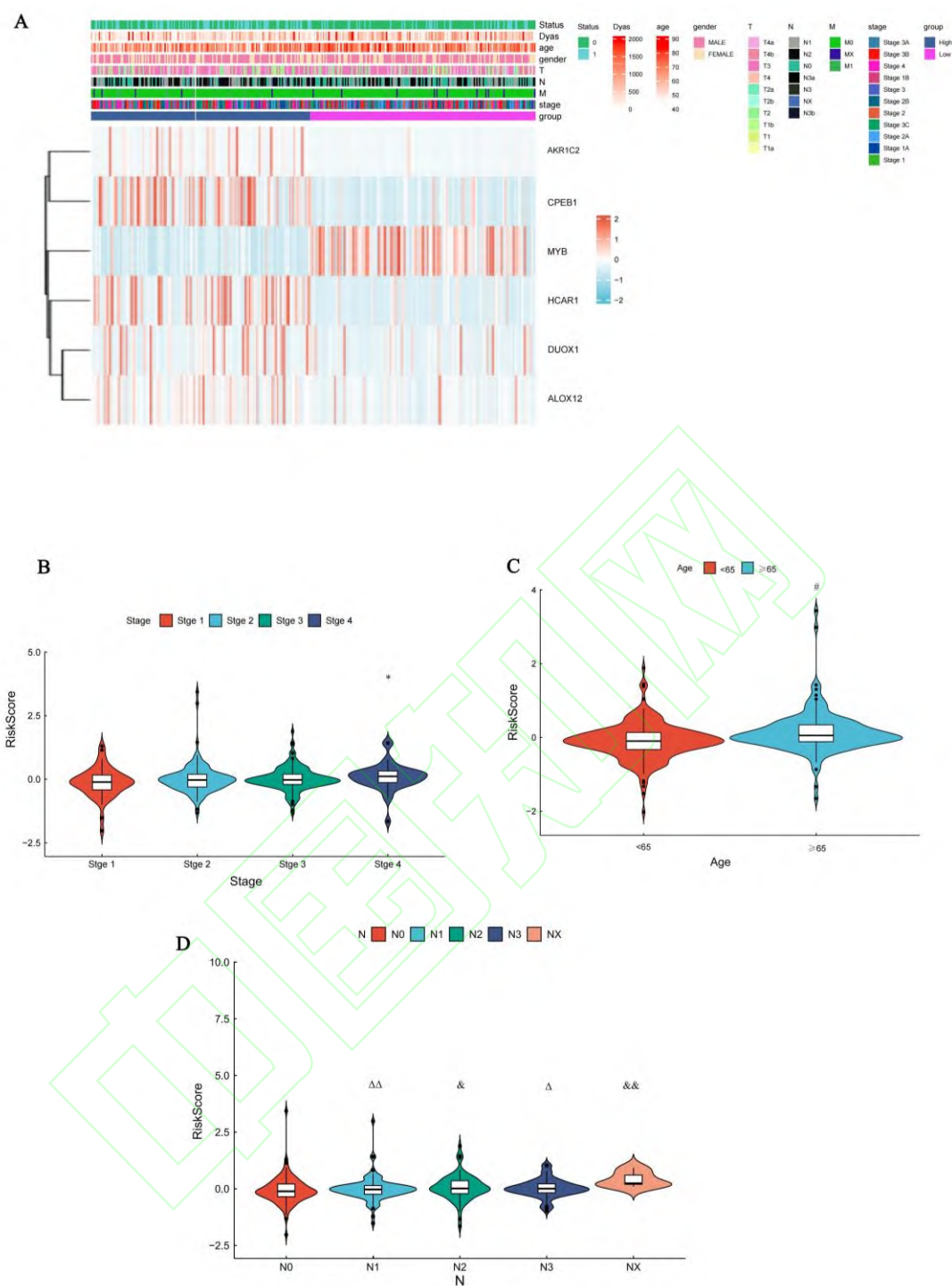
图 3 TCGA 数据库中预后特征与临床病理特征之间的相关性分析
