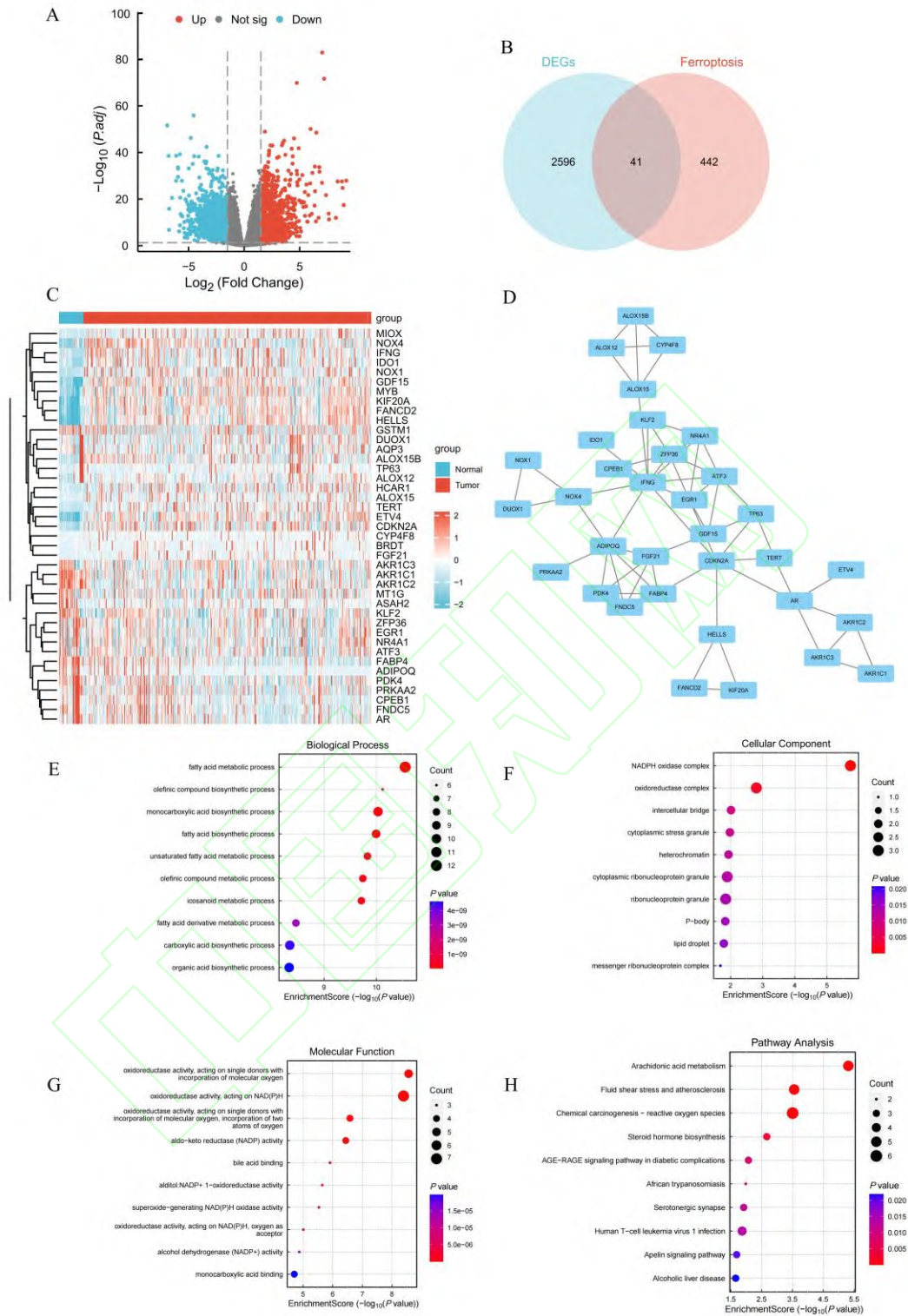
图 1 差异表达铁死亡相关基因的筛选和功能富集分析
