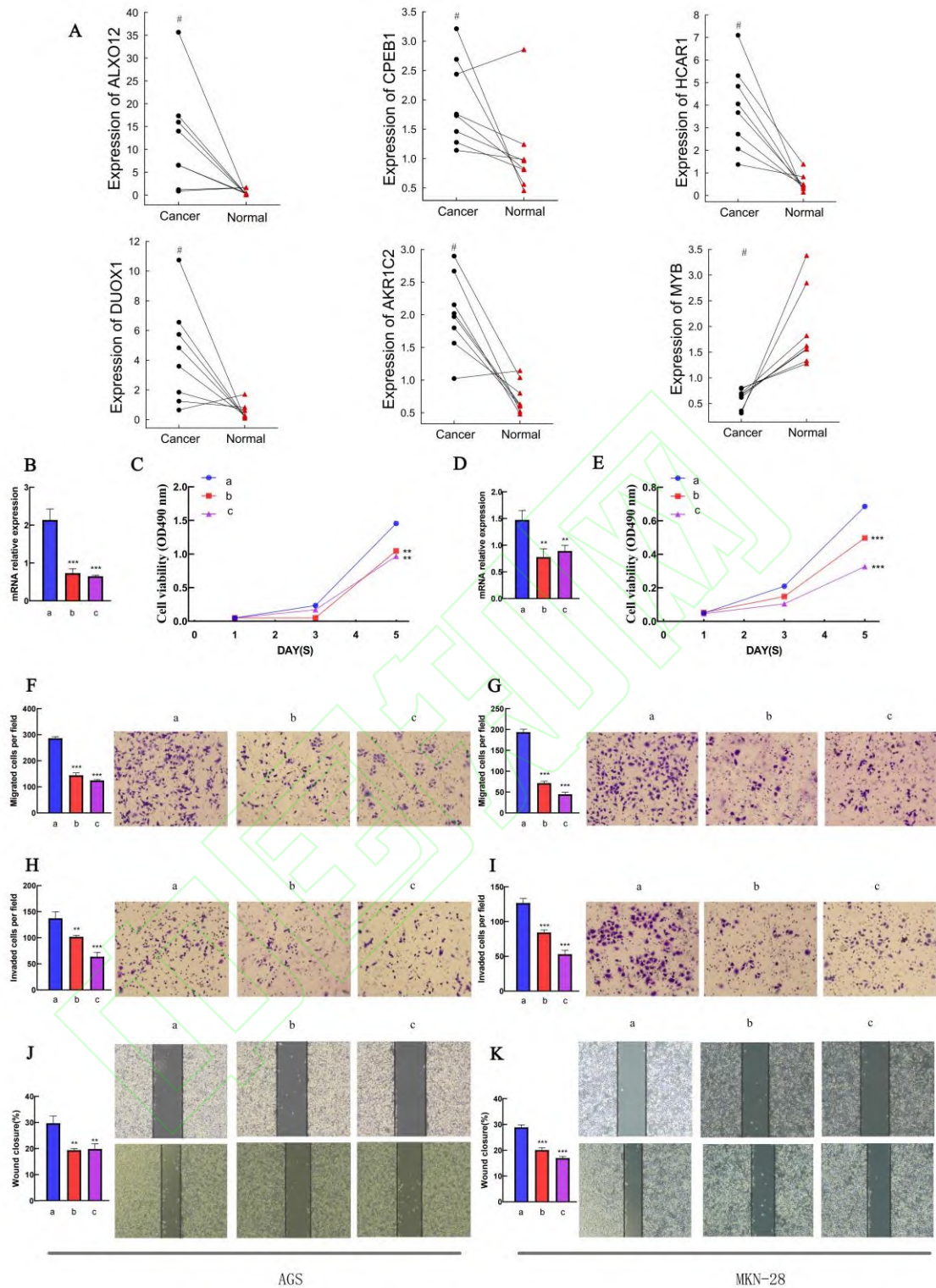
图 5 6 个关键基因在组织样品和 HCAR1 的体外功能实验验证
